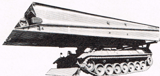
26 Brückenlegepanzer Biber mit beweglicher Brücke, Bundeswehr Char poseur pont, pont mobile, Allemagne Bridge layer „Beaver“ with movable bridge, Western Germany 2,95 DM
